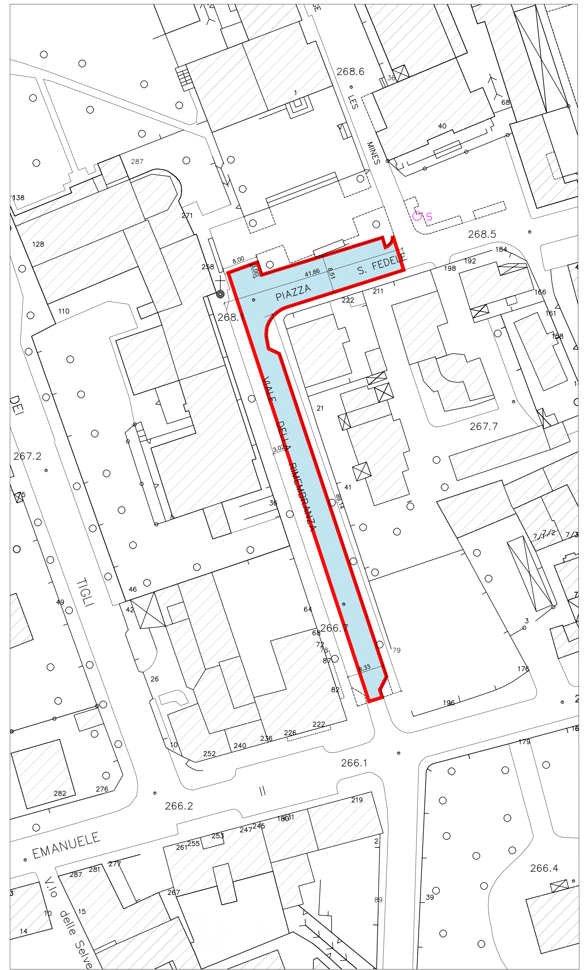
PROGETTO - PLANIMETRIA VIALE DELLE RIMEMBRANZE - SCALA 1:500
