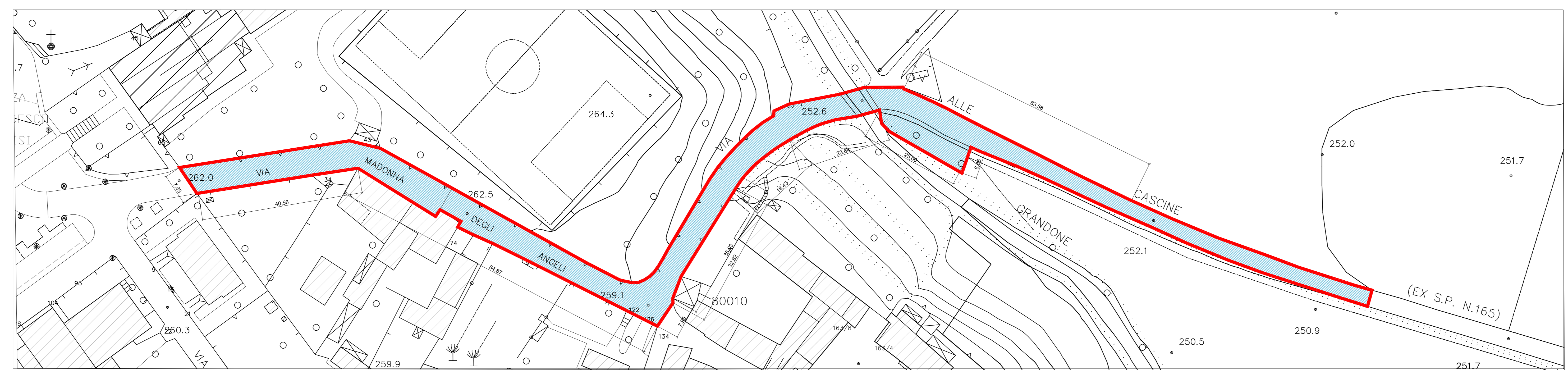
PROGETTO - PLANIMETRIA VIE MADONNA DEGLI ANGELI - DELLE CASCINE - SCALA 1:500
